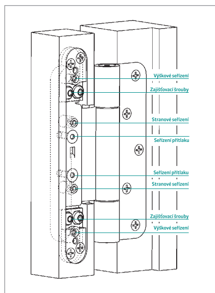
Tri-dimenzionální, plynulé seřízení. Všechny seřízení lze provést pomocí šestihybného klíče SW 4 mm
